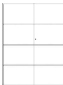
AC05 Dimensões L. 1200 x P. 420 x A. 1600 mm 3 prateleiras 4 espaços úteis
