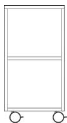
ND510 Dimensões L. 430 x P. 375 x A. 838 mm
