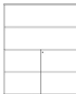
AC58 Dimensões L. 1200 x P. 420 x A. 1480 mm 3 prateleiras 4 espaços úteis
