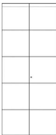
AL05 Dimensões L. 845 x P. 395 x A. 2030mm 4 prateleiras 5 espaços úteis
