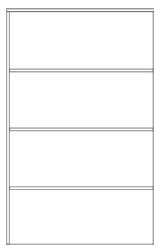
AC34 Dimensões L. 1000 x P. 420 x A. 1600 mm 3 prateleiras 4 espaços úteis
