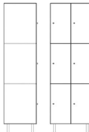
THP6 Dimensões L. 630 x P. 500 x A. 1980 mm
