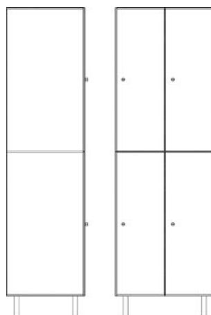
THP4 Dimensões L. 630 x P. 500 x A. 1980 mm
