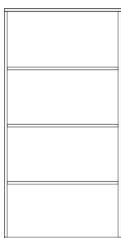
AC33 Dimensões L. 800 x P. 420 x A. 1600 mm 3 prateleiras 4 espaços úteis
