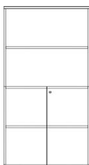
AC56 Dimensões L. 800 x P. 420 x A. 1480 mm 3 prateleiras 4 espaços úteis
