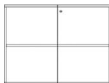
AC010 Dimensões L. 1000 x P. 420 x A. 740 mm 1 prateleira 2 espaços úteis
