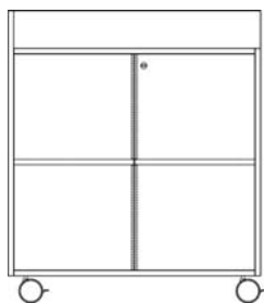
AR5L Dimensões L. 840 x P. 375 x A. 968 mm
