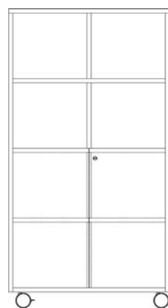
ND590 Dimensões L. 840 x P. 375 x A. 1567 mm
