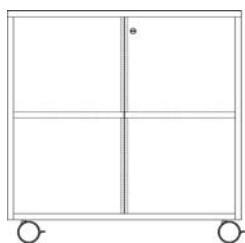
ND560 Dimensões L. 840 x P. 375 x A. 838 mm
