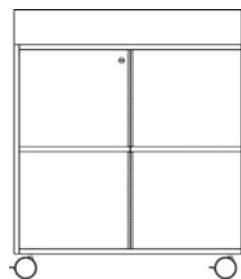
AR5R Dimensões L. 840 x P. 375 x A. 968 mm
