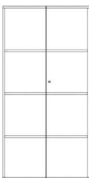
AC03 Dimensões L. 800 x P. 420 x A. 1600 mm 3 prateleiras 4 espaços úteis
