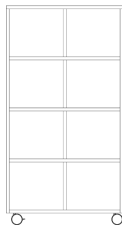
ND530 Dimensões L. 840 x P. 375 x A. 1567 mm
