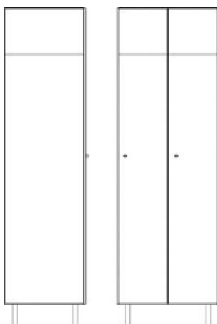
THP2 Dimensões L. 630 x P. 500 x A. 1980 mm
