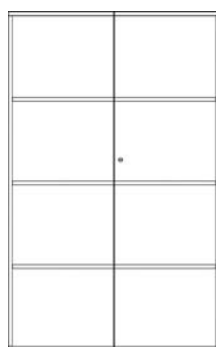
AC04 Dimensões L. 1000 x P. 420 x A. 1600 mm 3 prateleiras 4 espaços úteis
