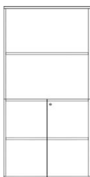
AC53 Dimensões L. 800 x P. 420 x A. 1600 mm 3 prateleiras 4 espaços úteis
